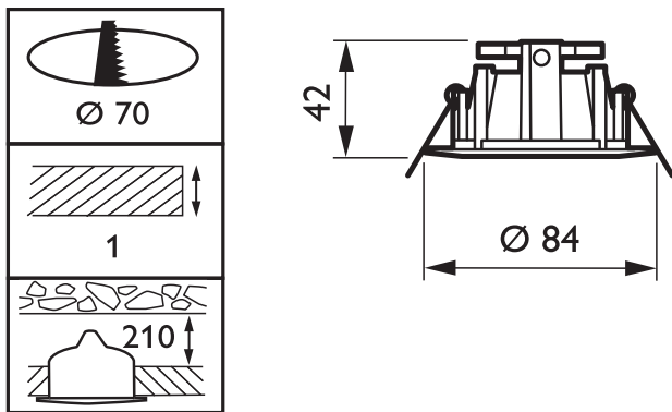
QBS023 1x MAX50W-GU5.3 12V WH
